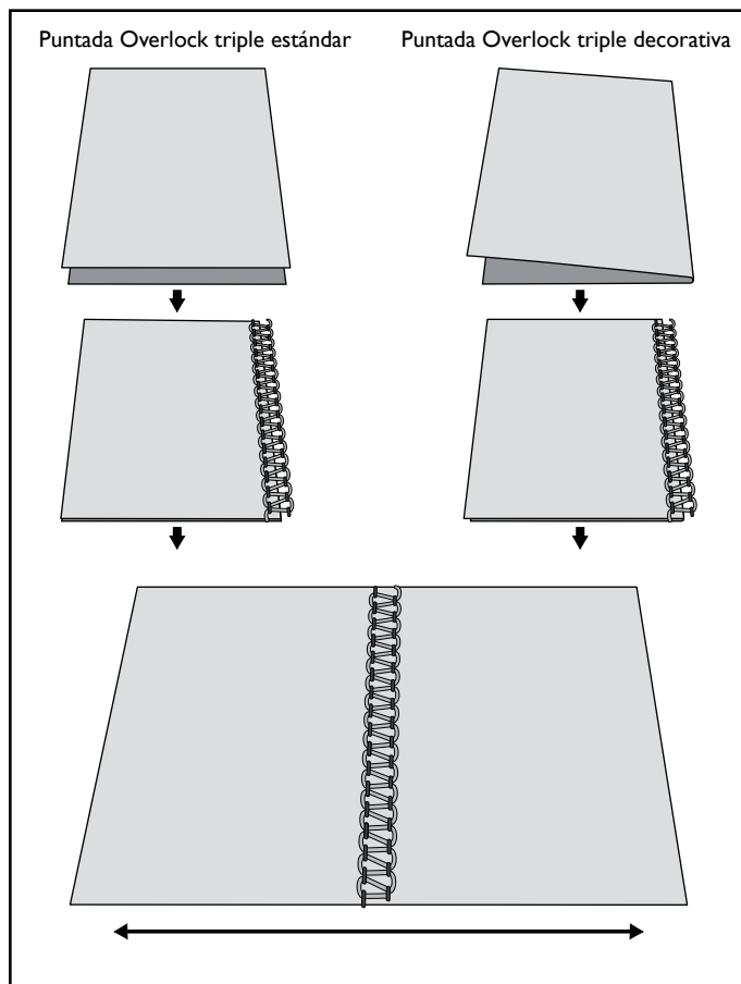
Puntada Overlock triple de dos hilos
